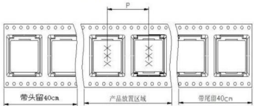
包装带尺寸图Tape size:
