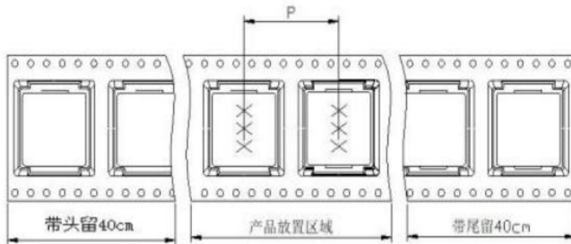
包装带尺寸图 Tape size:
