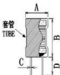
正视图 FRONT VIEW
