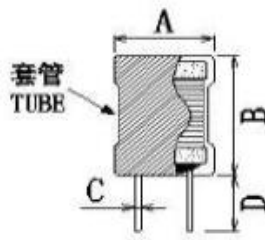
正视图 FRONT VIEW
