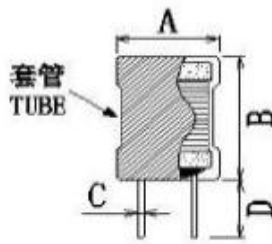
正视图 FRONT VIEW
